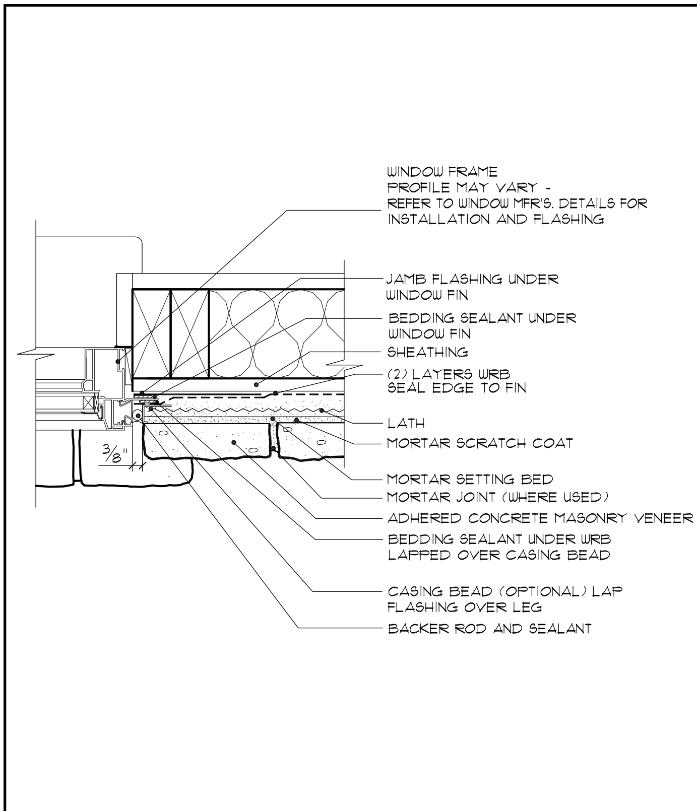
Fig. 20. Window Jamb
