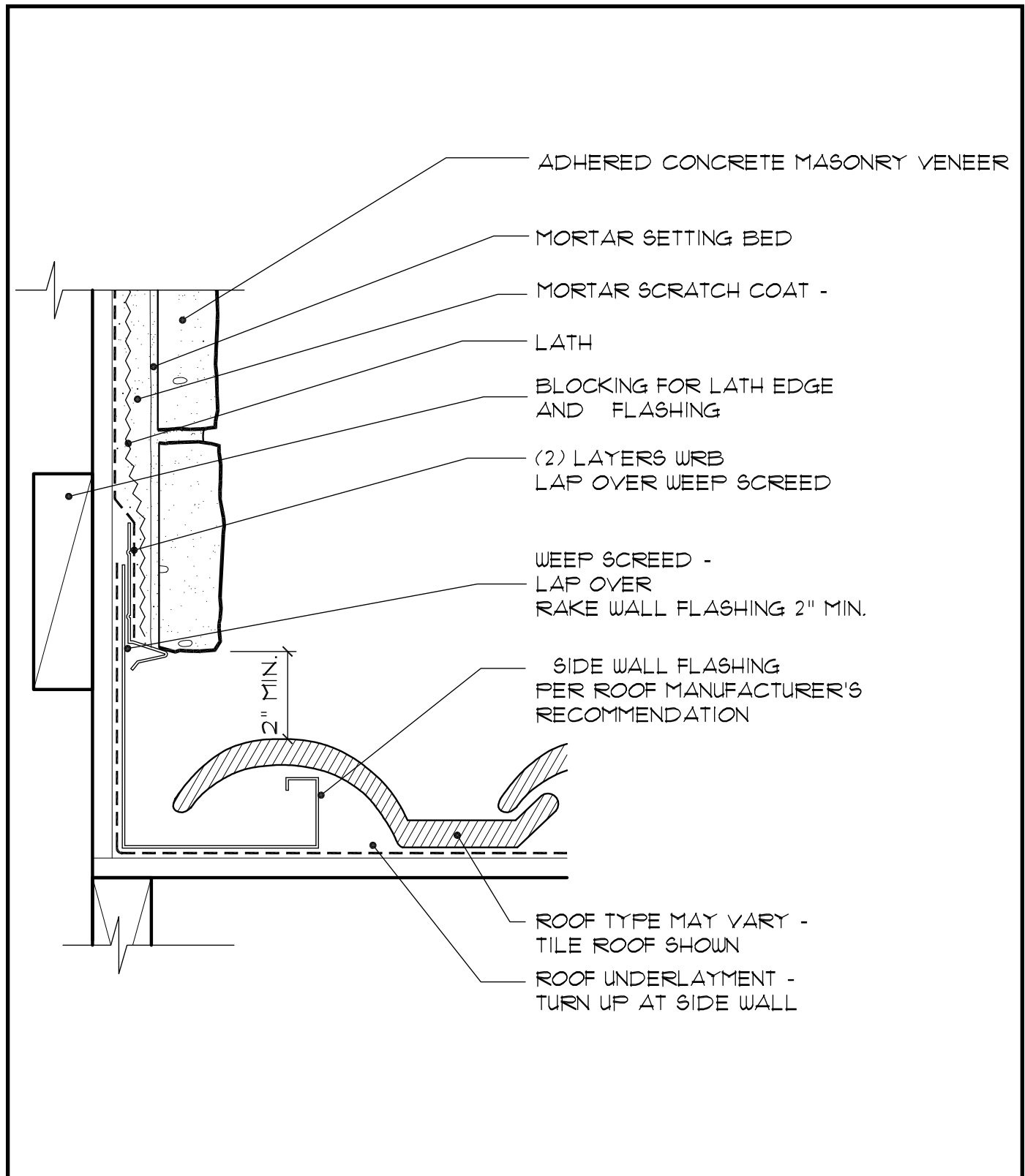
Fig. 17. Side Wall - Tile Roofing
