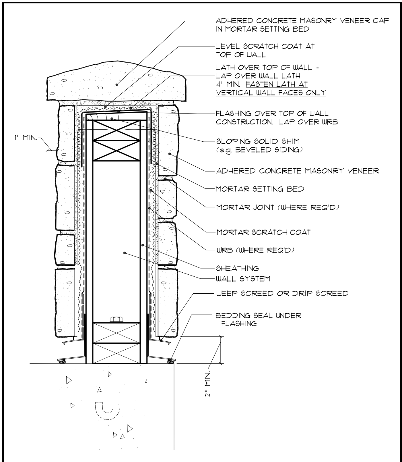
Fig. 33. Wall Cap
