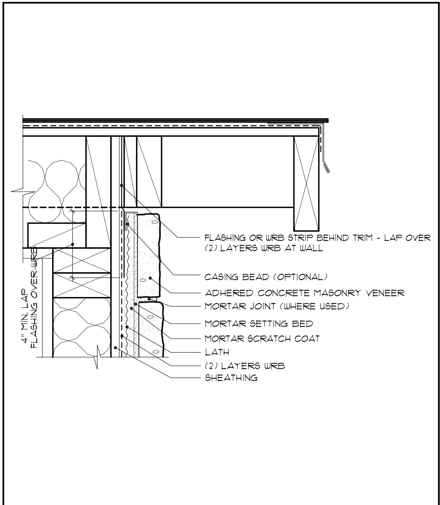
Fig. 13. Rake - Overhang
