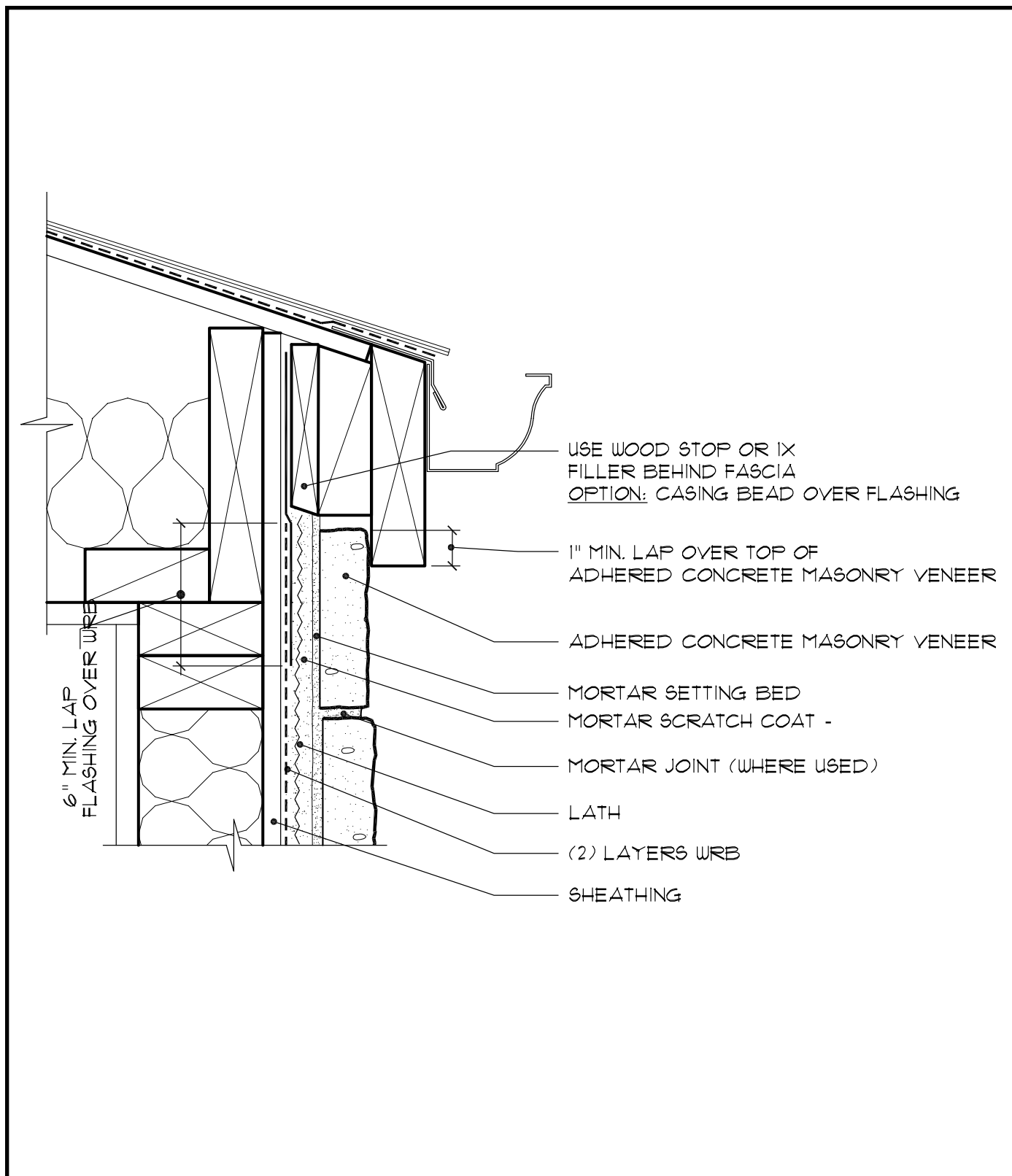
Fig. 12. Open Eave - Flush
