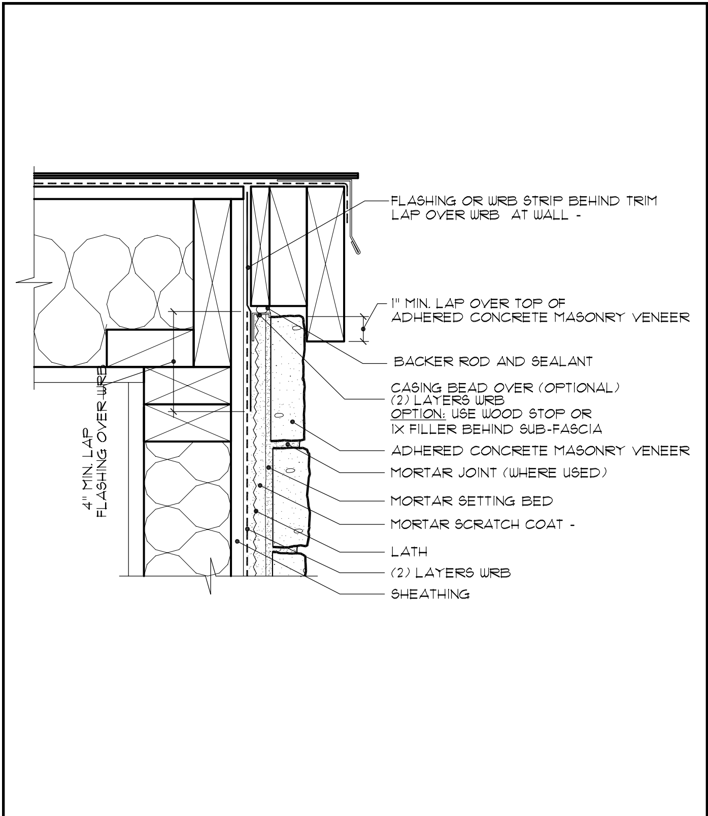
Fig. 14. Rake - Flush
